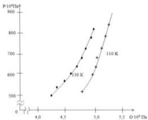
№9 сызба. Ih мұз модификациясының әртүрлі
